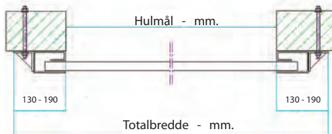
Vandret snit
